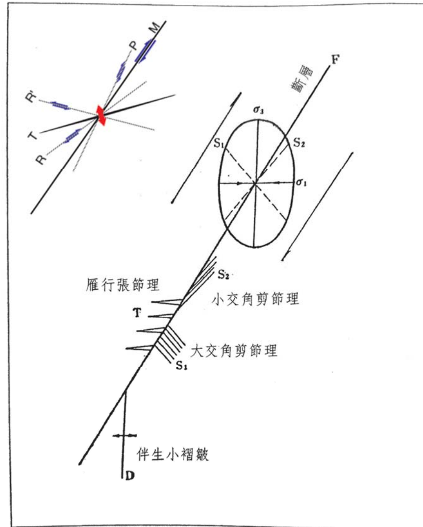
圖 8.18 與斷層伴生的雁行節理及小褶皺
