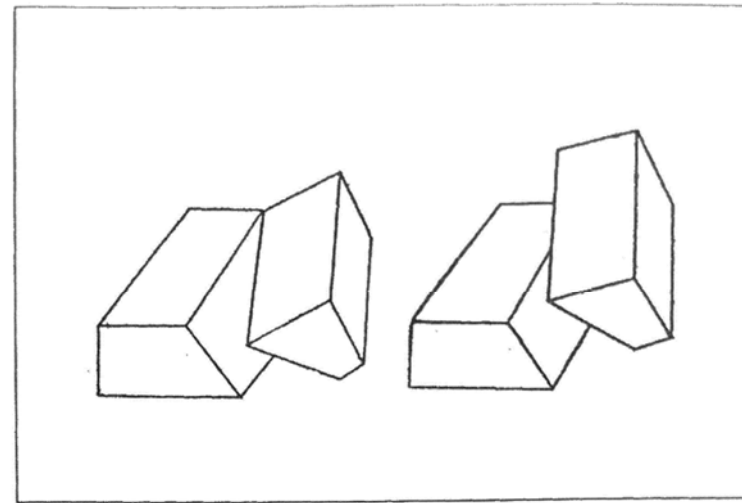
圖 8.11 斷層的旋轉運動
