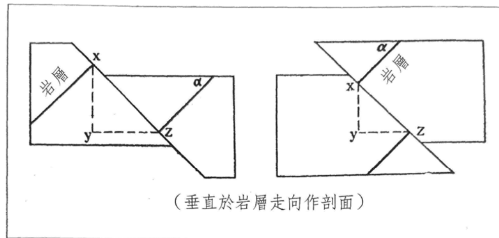
圖 8.6 岩層的落差 (xy) 及平錯 (yz)
