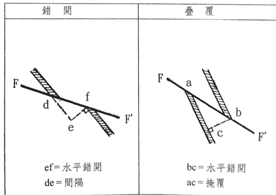
圖 8.7 岩層的錯開與掩覆
