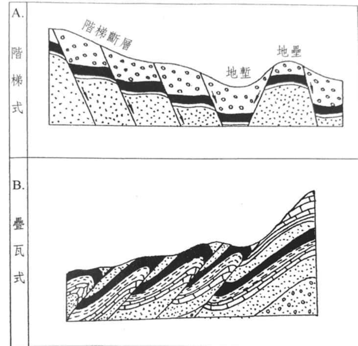
圖 8.13 幾種常見的斷層組合型態
