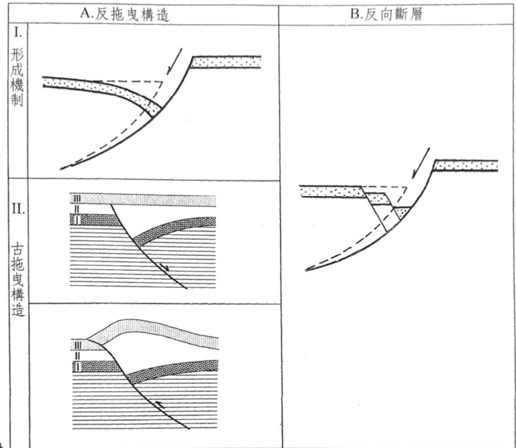
圖 8.17 反拖曳構造與反向斷層
