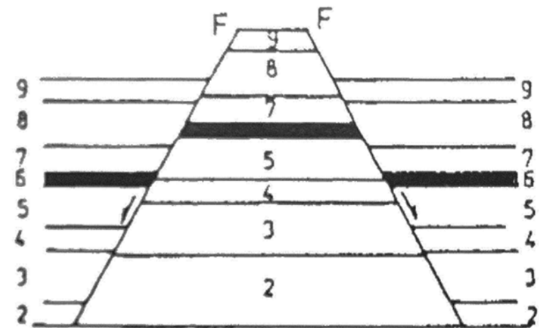
(b)地隆 (或譯地壘)
