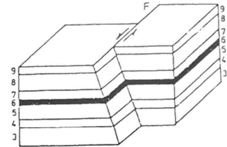
(d) 平移斷層 (Strike-Slip Fault)
