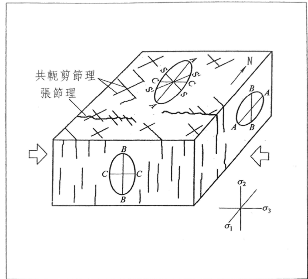
圖 8.2 應變橢圓球的應用
