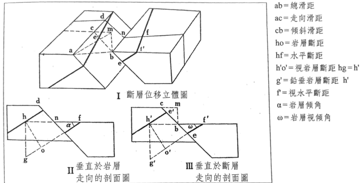
圖 8.5 斷層的滑距及斷距
