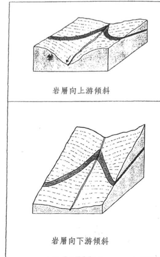
圖 7.7 V 字型露頭線指向上游，岩層可能向上游傾斜，也可能向下游傾斜
