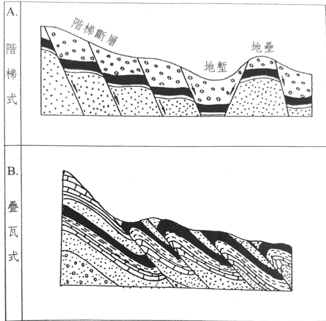
圖 8.13 幾種常見的斷層組合型態
