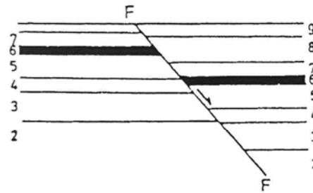
(b) 正斷層 (Normal Fault)
