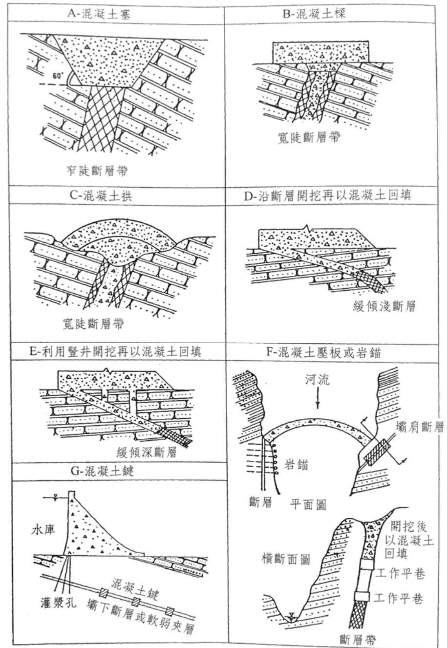
圖 8.28 斷層帶的各種處理方法 (張咸恭等, 1988)
