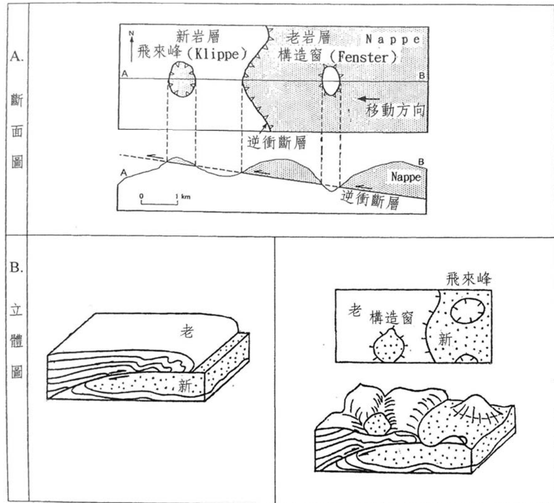
圖 8.10 構造窗及飛來峰的形成發育過程
