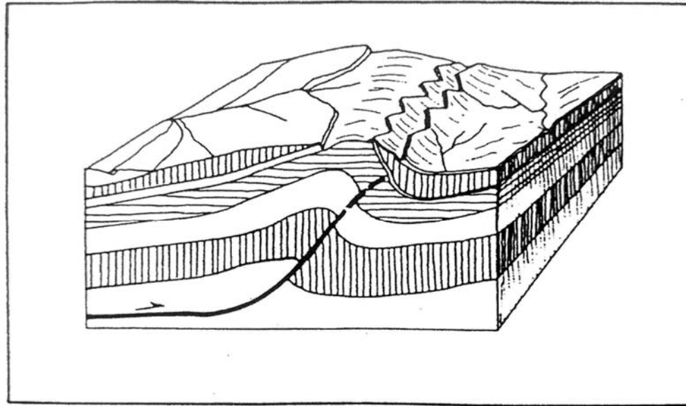
圖 7.8 岩層三角面
