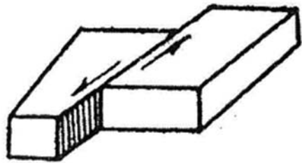
平移斷層
