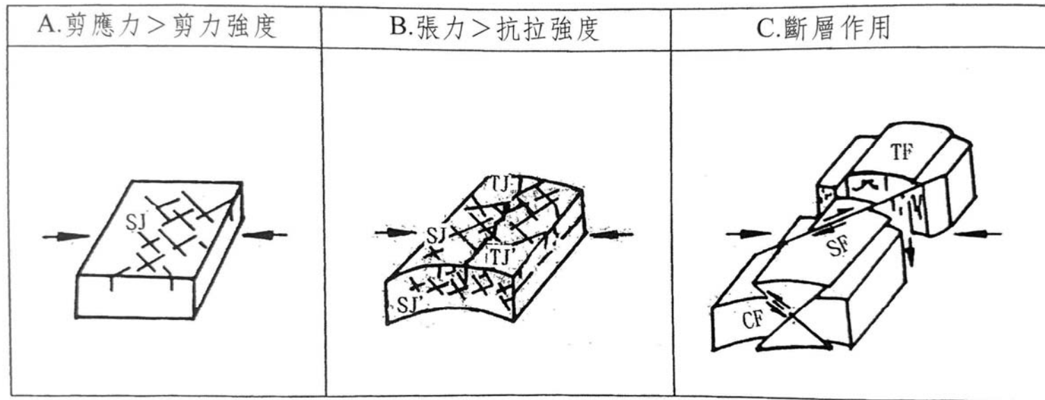
圖 8.3 斷裂構造的形成過程
