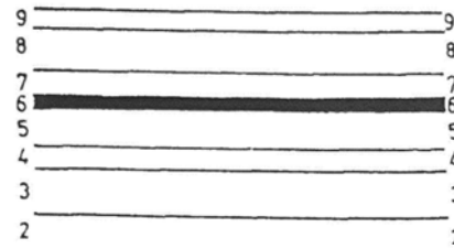
(a) 沈積岩在未發生斷層前之剖面
