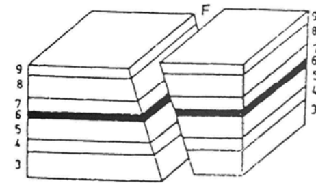
(f) 斜移斷層 (Oblique-Slip Fault)
