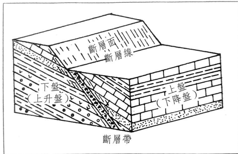
圖 8.4 斷層的幾何要素
