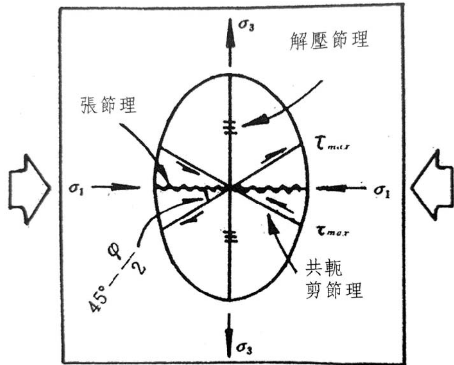
圖 8.1 應變橢圓球與斷裂構造的關係
