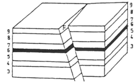
(e) 鉸移斷層 (Hinge Fault)
